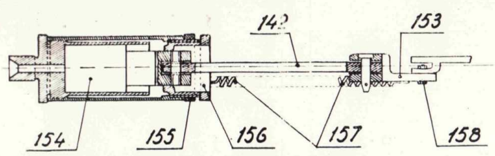
Spust pneumatyczny k.m. skrzydł.
